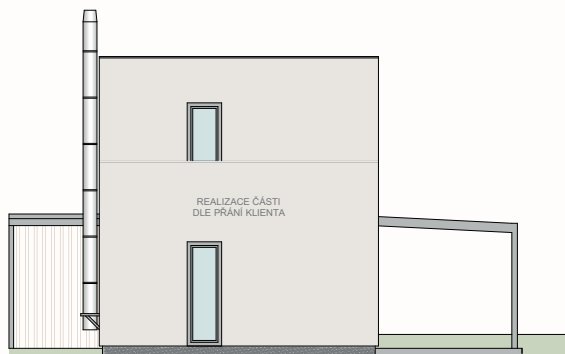
FASÁDA SEVEROVÝCHODNÍ
