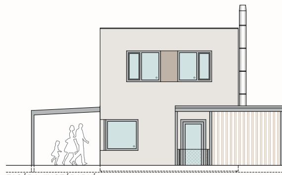
FASÁDA JIHOZÁPADNÍ
